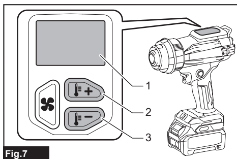
► 1. Pantalla de estado 2. Botón más (+) de ajuste de temperatura 3. Botón menos (-) de ajuste de temperatura
