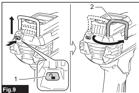
► 1. Botón de liberación de gancho 2. Gancho
